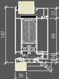
Montage: außen bündig
