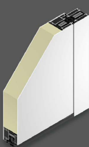
Außenansicht flügelüberdeckend
