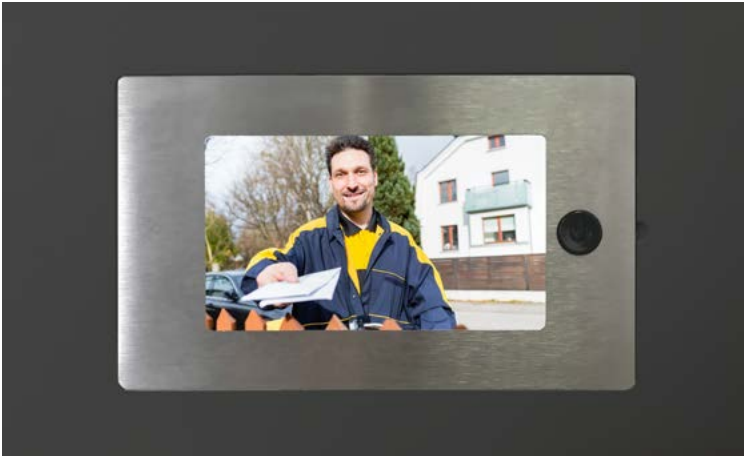
Digitaler Türspion hoch auflösender LCD-Bildschirm, flächenbündig im Türblatt integriert inkl. Magnethaltung (nur bei beidseitig flügelüberdeckender Ausführung möglich)
