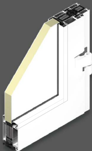
Innenansicht Glasfalz mit Standard-Aufsatztürbändern
