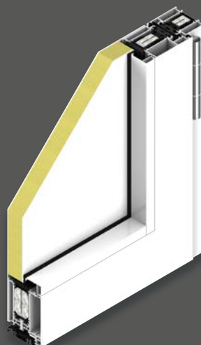
Innenansicht Glasfalz mit Rollentürbändern
